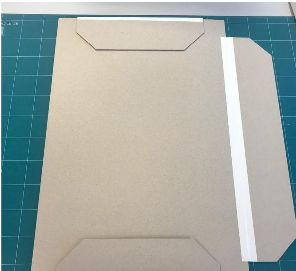
Zdjęcie 15. Fotografia przedstawia przyklejone na taśmę płócienną tekturowe listwy.
