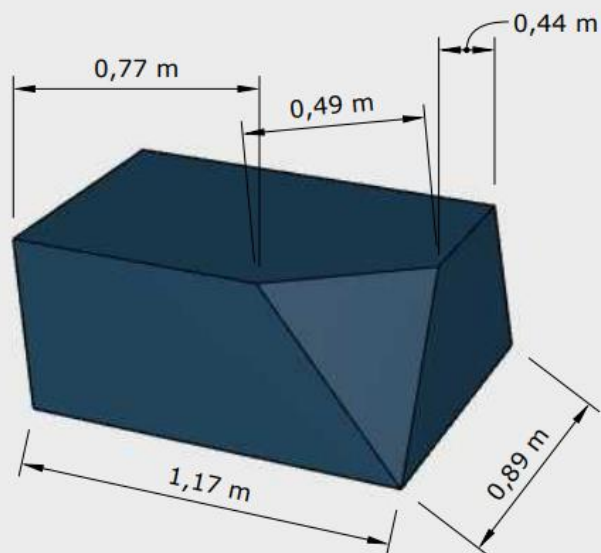
KUBIK NIEBIESKI RZUT IZOMETRYCZNY 3
