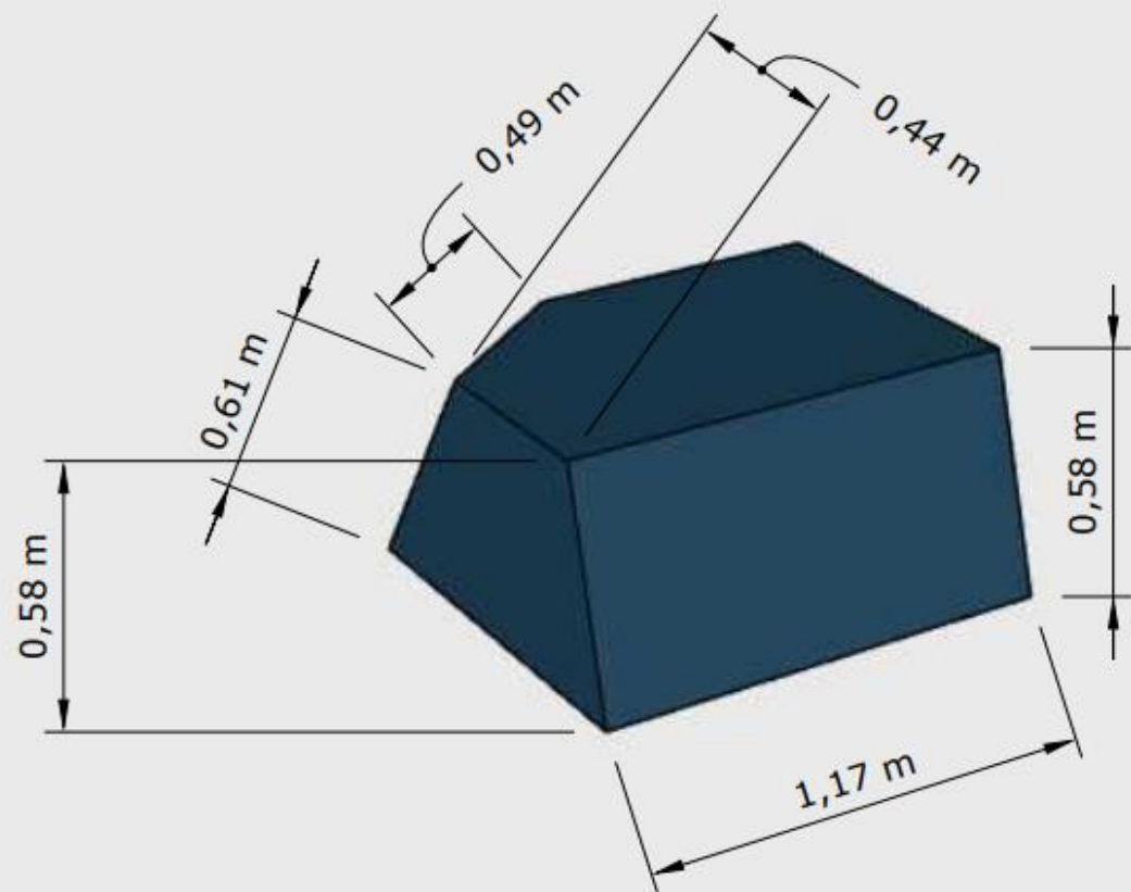
KUBIK NIEBIESKI RZUT IZOMETRYCZNY 2
