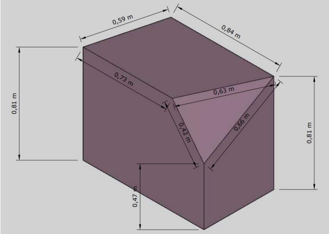
KUBIK WRZOSOWY RZUT IZOMETRYCZNY 1
