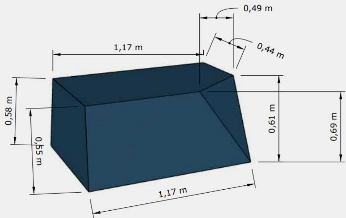
KUBIK NIEBIESKI RZUT IZOMETRYCZNY 1
