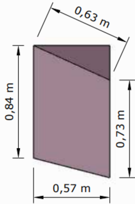
KUBIK WRZOSOWY RZUT Z GÓRY
